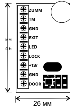
Рис.1 Зовнішній вигляд і габаритні розміри плати
