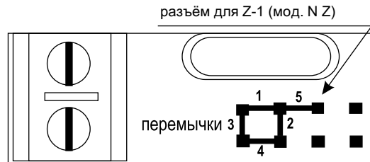
Рис. 2 Положення перемичок
