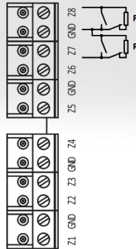
Рис.14. Підключення шлейфів блокування та вільного проходу
