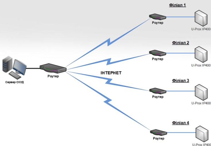
Рис. 4. Приклад розподіленої мережі
