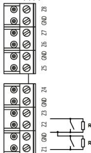
Рис.11. Підключення кнопки запиту проходу
