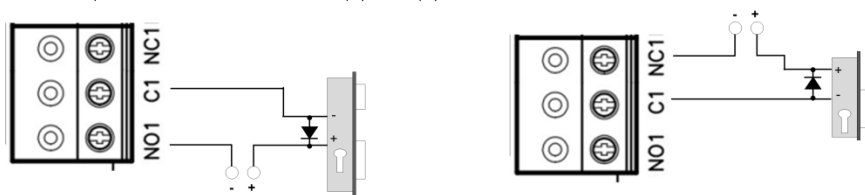
Рис.15. Підключення замків під час використання зовнішнього джерела живлення
