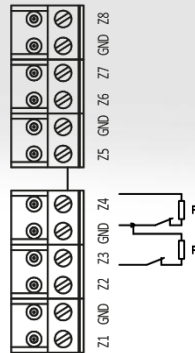
Рис.12. Підключення дверного контакту
