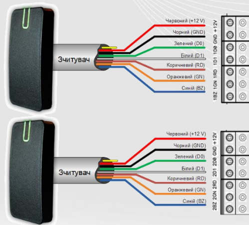
Рис.10. Підключення зчитувачів
