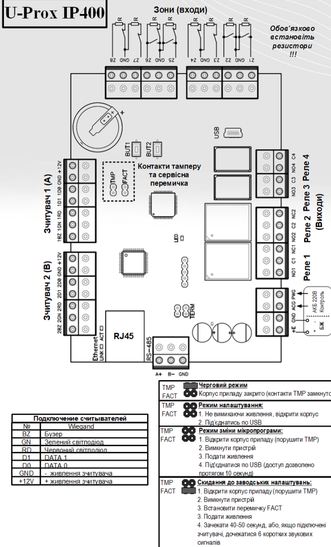
Рис. 2. Зовнішній вигляд плати контролера
