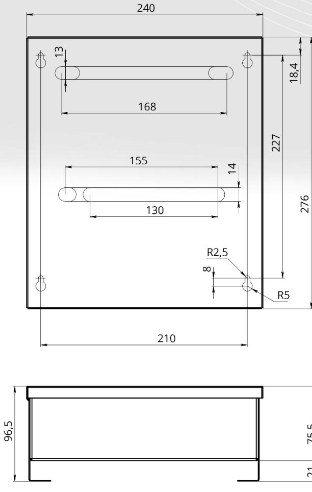
Рис. 9. Габаритні розміри та розмітка отворів кріплення
