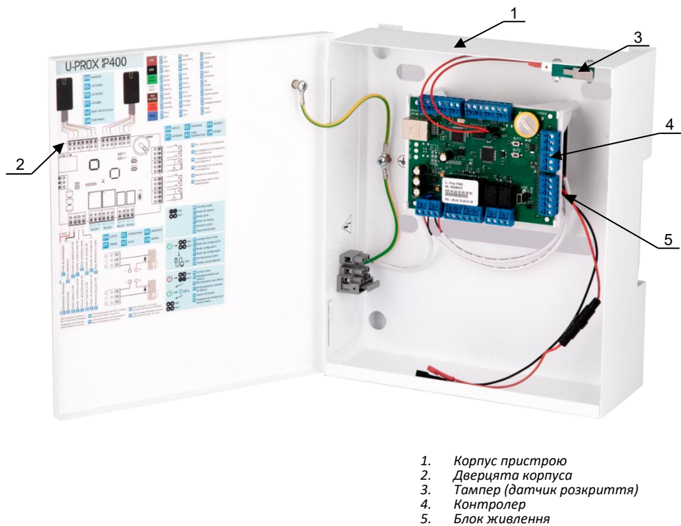
Рис. 1. Зовнішній вигляд U-PROX IP400
