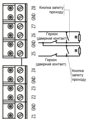
Рис.13. Підключення комбінованого шлейфу
