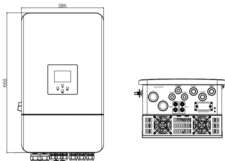
Розмір інвертора
