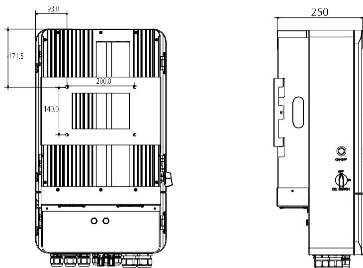
Розмір інвертора
